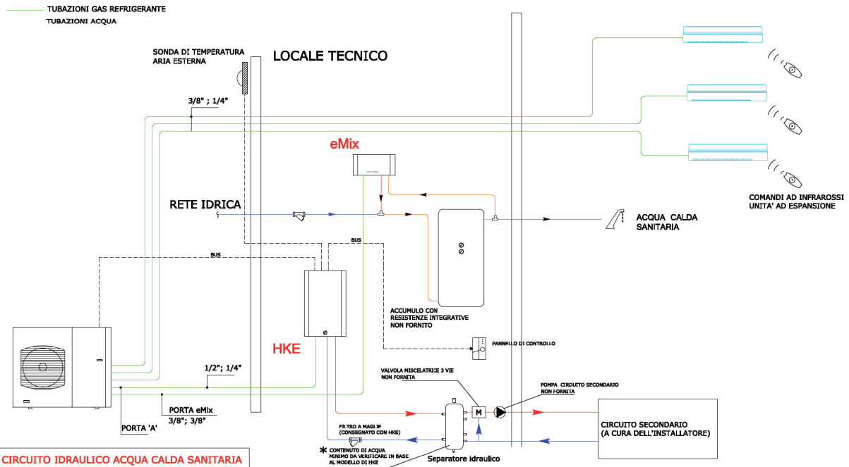
CIRCUITO IDRAULICO ACQUA CALDA SANITARIA
